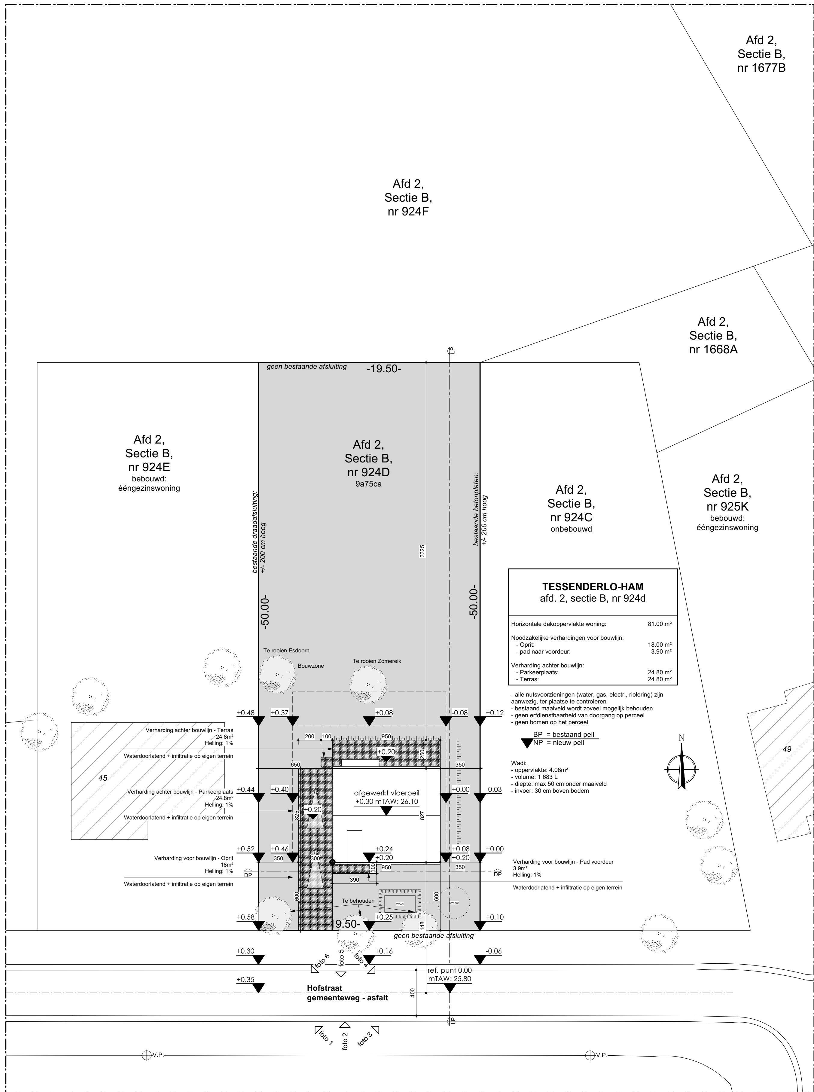
I Inplantingsplan Schaal: 1:200
