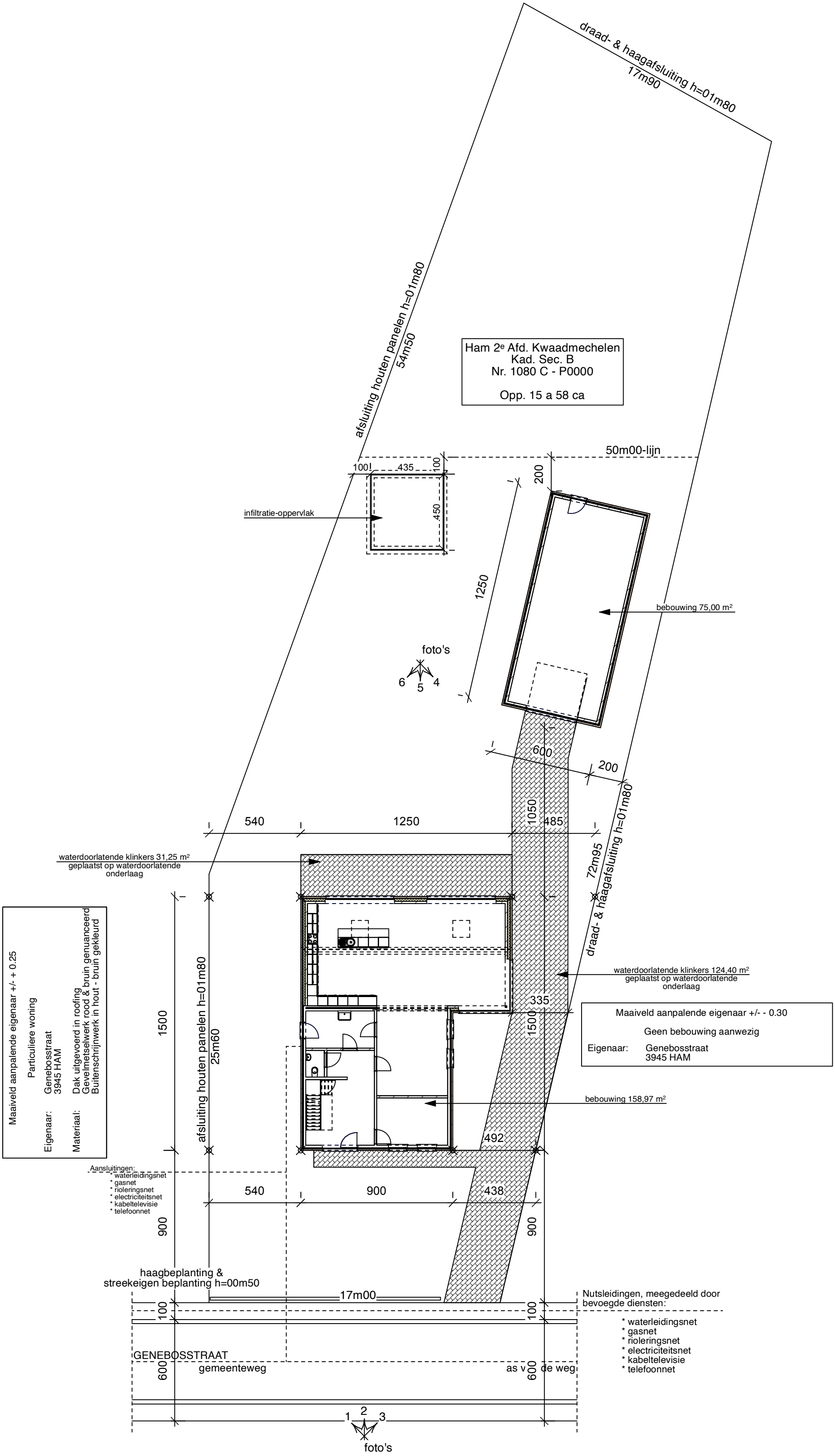
INPLANTINGSPLAN (schaal 1/200)
